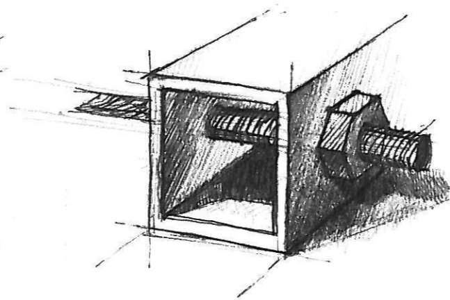
Acelsodrony csatlakozása a zártszelvényhez
