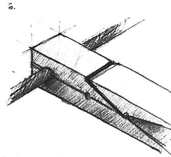
Csiperz csatlakozása a sodronyhoz
