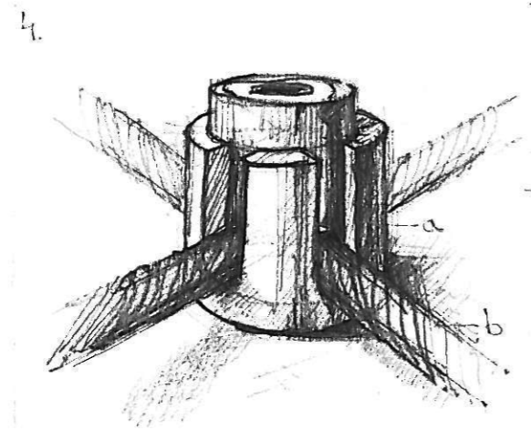
Sodronykeresztvázas rögzítése a) Sodronykeresztvázas rögzítés - 1560 db - 20 Ft/db b) Horgonyzott sodronyöbél - 1060 m - 39 Ft/m
