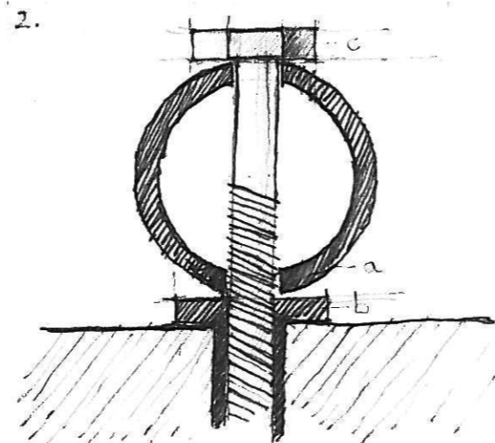
Cső leforgatása a padlózatba féműrtéssel a) Cső - 24 fm - Ø 1" - 2.500 Ft/m b) Féműrtével - ME - 13 Ft/db c) Fémcsavar - ME * 60 - 9 Ft/db
