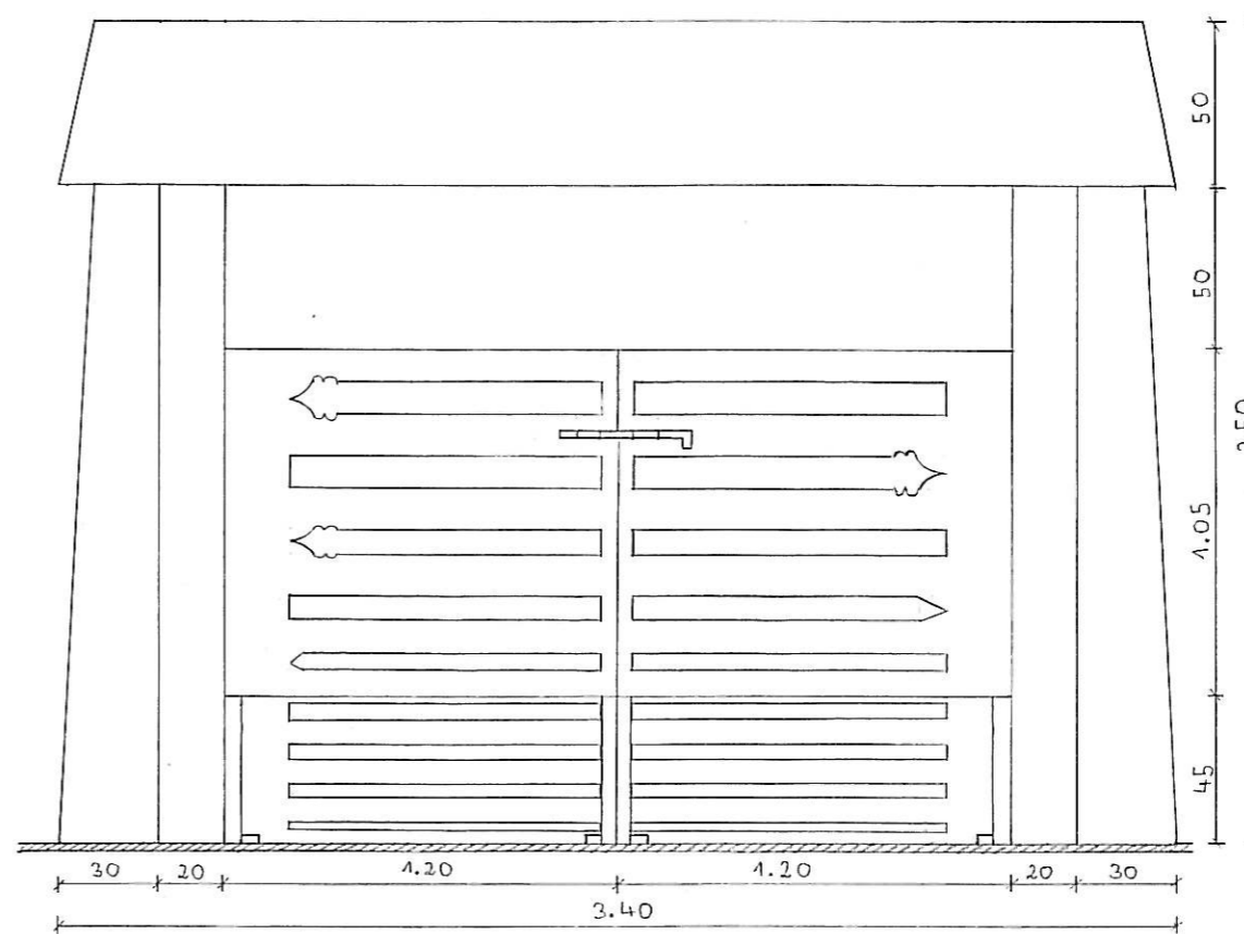
KAPU HÁTULNÉZET
