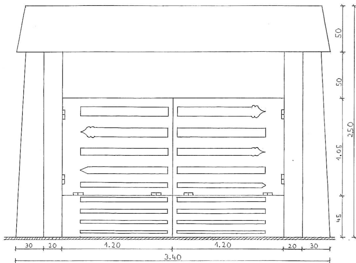
KAPU ELŐNÉZET
