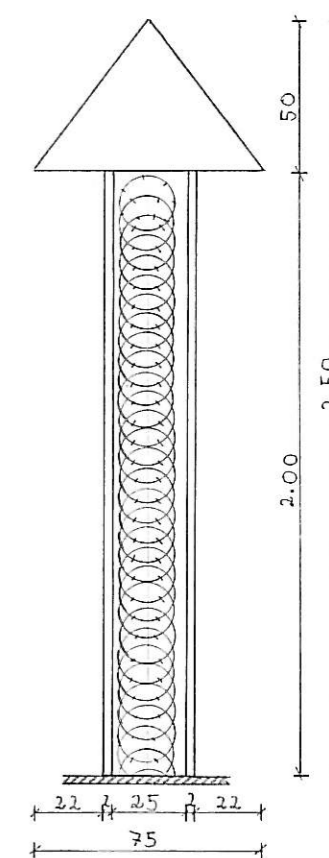
KAPU OLDALNÉZET
